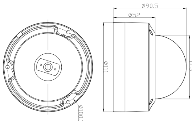
Рисунок А.26 – Габаритный чертеж видеокамеры ИВМ-401.
